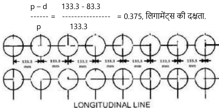
चित्र 4/8 - प्रत्येक पंक्ति में समान छेद की पिच के साथ ट्यूबों की दूरी का उदाहरण पंक्ति
