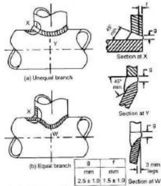
चित्र 12/118: बैकिंग के बिना समकोण शाखाओं पर सेट हेतु विशिष्ट तैयारी और असेंबली
