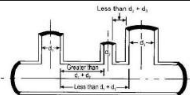
चित्र 7/8 : विशिष्ट ब्रांच के टुकड़े
