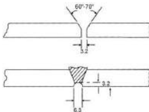
चित्र 2/6: बैकिंग रन के डिसपोजीशन के लिए प्रिपरेशन में ग्राविंग
