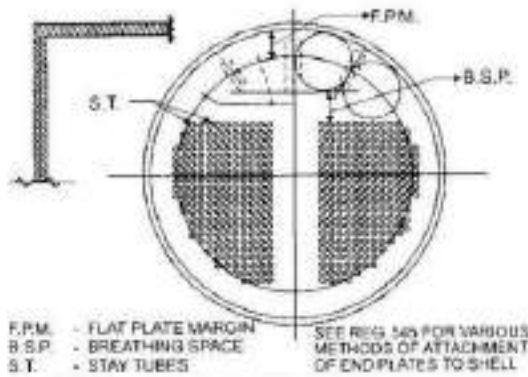
चित्र 12/93: मल्टी ट्यूबलर बॉयलर पर एंड प्लेट का टिपिकल अरेंजमेंट
