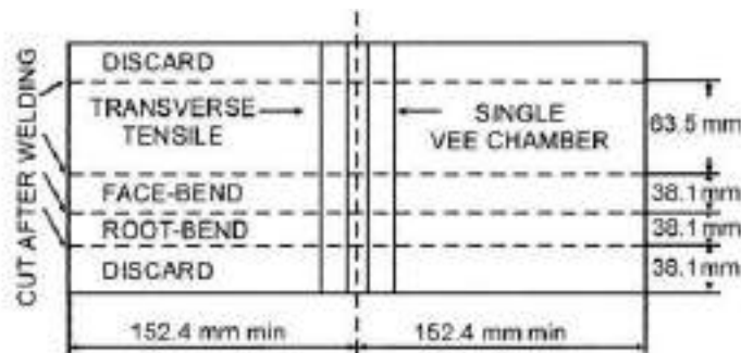
चित्र 2/5: ट्रांसवर्स तन्यता और बेंड परीक्षण नमूने तैयार करने की पद्धति
