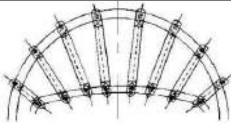
चित्र 12/93: मल्टी ट्यूबलर बॉयलर पर एंड प्लेट का टिपिकल अरेंजमेंट
