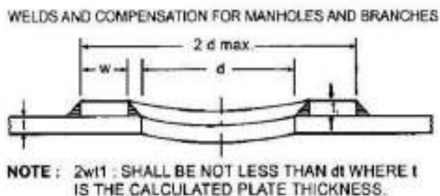
चित्र. 10/9 : बाहरी क्षतिपूर्ति रिंग
