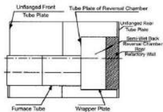
चित्र 12/27: सेमी-वेट बैक बॉयलर
