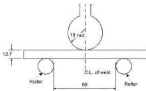
चित्र. 2/8: बेंड परीक्षण करने की पद्धति
