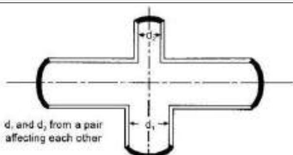
चित्र 7 /6 : विशिष्ट ब्रांच के टुकड़े
