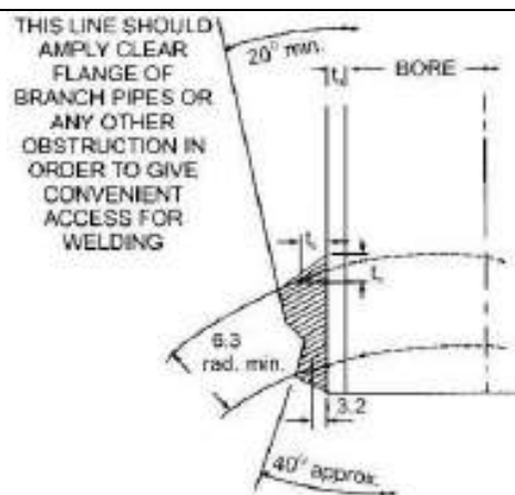
चित्र 4/31: स्टैंडपाइप या ब्रान्च में वेल्ड किया
