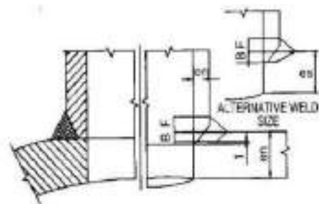
चित्र 4/36: शेल के भीतर वेल्डिंग के लिए दुर्गम अप्रतिबंधित ब्रांचेज
