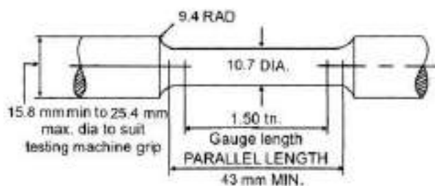
चित्र 2/3: तन्यता परीक्षण नमूना
