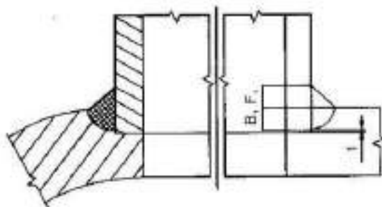
चित्र 4/35: शेल के भीतर वेल्डिंग के लिए दुर्गम अप्रतिबंधित ब्रांचेज
