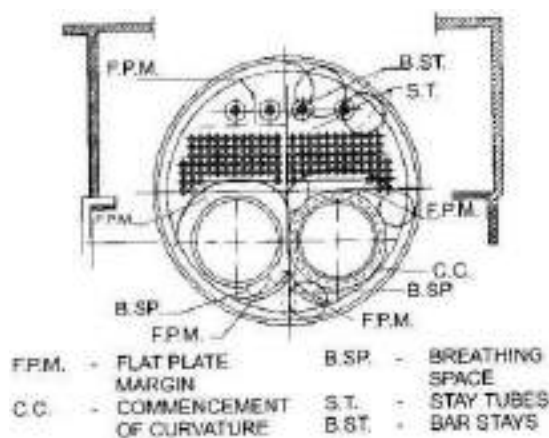
चित्र 12/91*: इकोनॉमिक बॉयलर का एंड प्लेट का टिपिकल अरेंजमेंट
