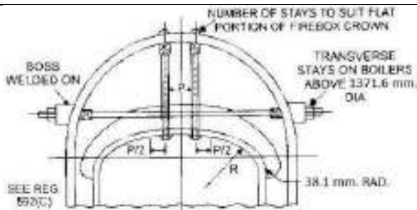
चित्र 12/95: लोकोटाइप बॉयलर के लिए फायर बॉक्स क्राउन और ट्रान्सवर्स स्टे की व्यवस्था
