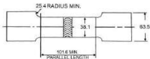
चित्र. 2/7: ट्रांसवर्स तन्यता परीक्षण नमूने का परिमाण
