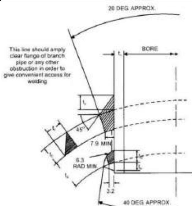
चित्र 4/26: स्टैंडपाइप या 101.6 मिमी बोर सहित स्टैंडपाइप या ब्रान्च में वेल्ड ब्रान्च के लिए प्रतिपूर्ति रिंग के साथ
