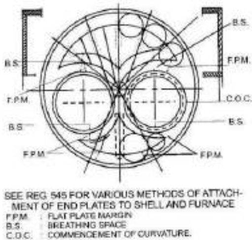
चित्र 12/87: लंकाशायर बॉयलर पर एंड प्लेट का टिपिकल अरेंजमेंट
