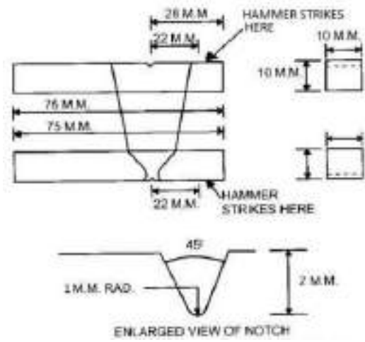
नमूना (2) और (3) प्रभाव परीक्षण
