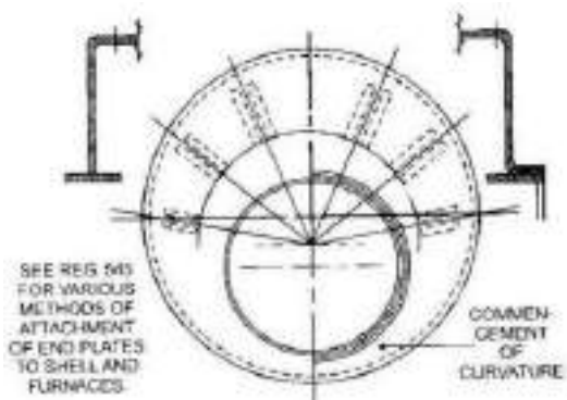
चित्र 12/88: कॉर्निश बॉयलर पर एंड प्लेट का टिपिकल अरेंजमेंट
