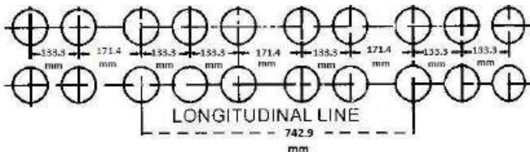
चित्र 4/10 - दूसरी और तीसरी पंक्ति में अलग-अलग छिद्रों की पिच के साथ ट्यूब स्पेसिंग का उदाहरण
