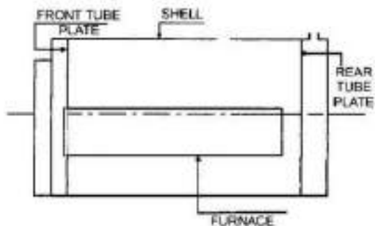
चित्र 12/24: रिवर्स फायर बॉयलर
