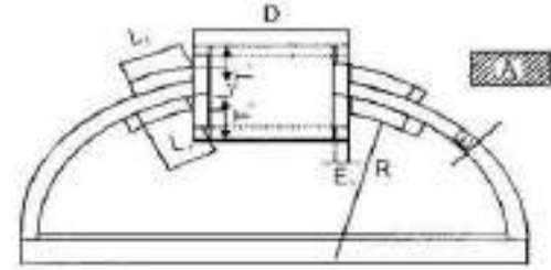
चित्र. 4/20: रीइन्फोर्स ओपनिंग
