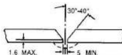
चित्र 7 / 11 : बैंकिंग रिंग के साथ उपयोग के लिए प्लेन वी
