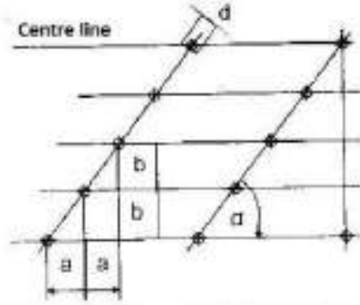
चित्र 4/14: छिद्रों का नियमित सॉ-टूथ पैटर्न
