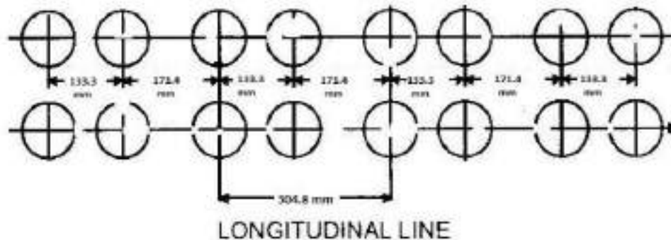
चित्र 4/9 - प्रत्येक पंक्ति में असमान छिद्रों की पिच के साथ ट्यूब स्पेसिंग का उदाहरण
