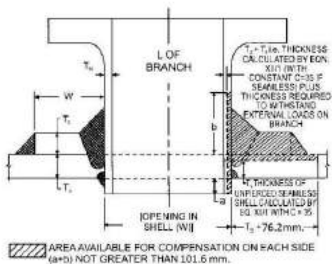
चित्र 12/80: ब्रांच के लिए कंपेंसेशन
