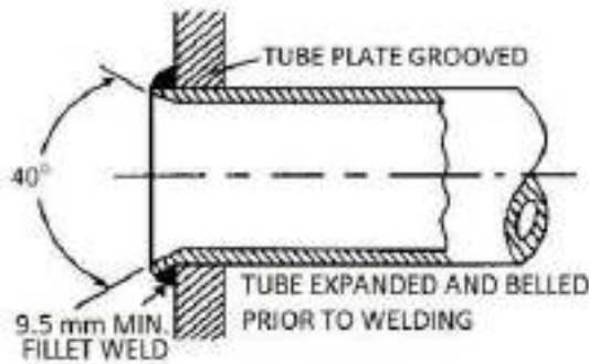
चित्र 3/10 वेल्ड स्टे ट्यूब का आदर्श उदाहरण
