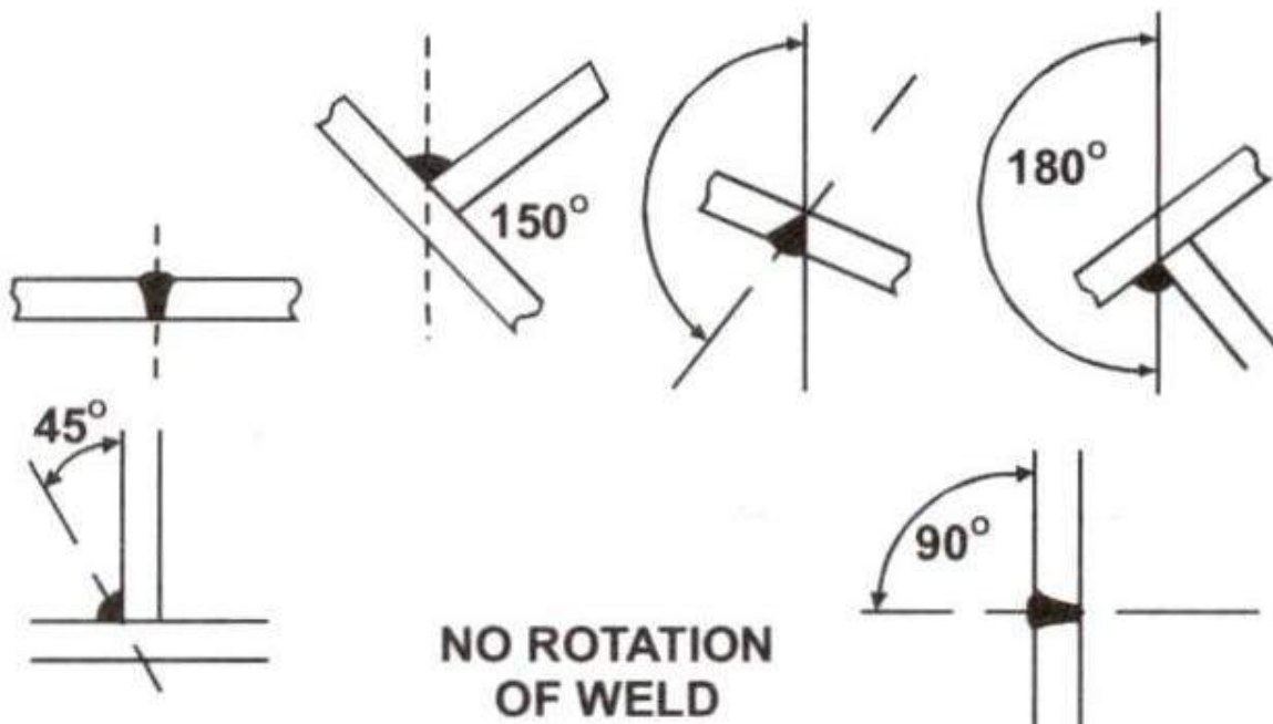
चित्र 2/10 : वेल्ड रोटेशन को दर्शाने वाले चित्र
