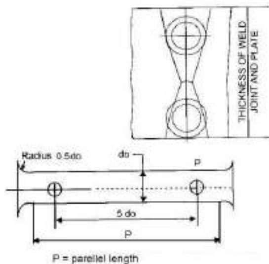
चित्र 12/77: टेंसाइल टेस्ट ऑल वेल्ड मेटल
