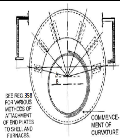
चित्र 12/89: कॉर्निश बॉयलर पर एंड प्लेट का टिपिकल अरेंजमेंट
