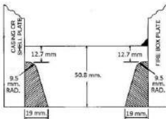
चित्र 12/37: फाउंडेशन रिंग्स
