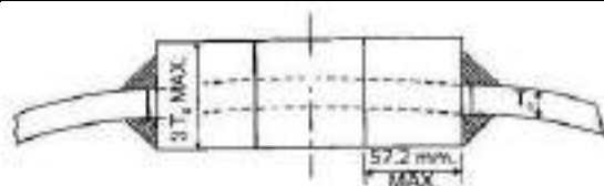
चित्र 12/115: स्टडस के लिए वेल्डेड पैड्स
