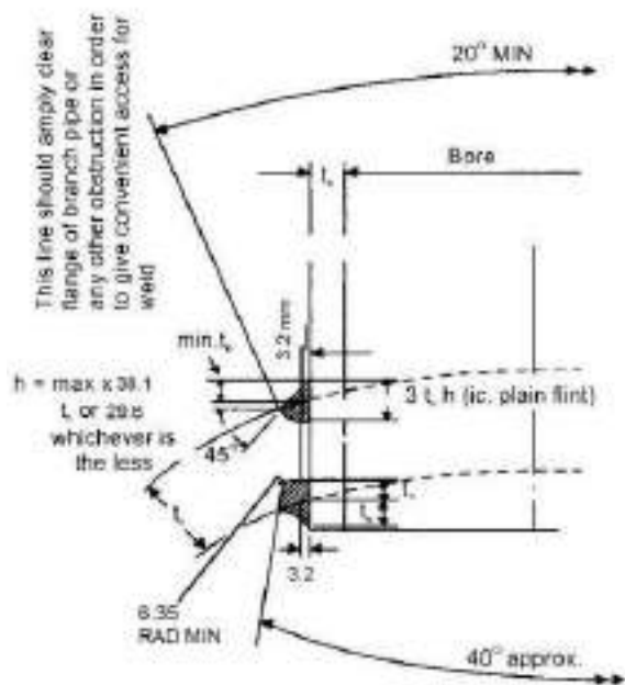
चित्र 4/25: स्टैंडपाइप या ब्रान्च या किसी भी ब्रान्च तक वेल्ड किया और 101.6 मिमी बोर सहित
