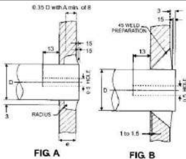
चित्र 12/50: फायरबॉक्स और रिवर्सल चैंबर का अटैचमेंट
