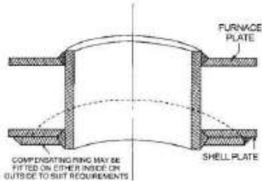
चित्र 12/40: फायरहोल माउथपीस
