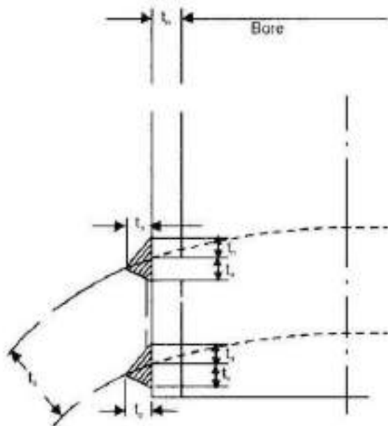
चित्र 4/24: स्टैंडपाइप और ब्रान्चों तक एवं 101.6 मिमी बोर सहित वेल्ड किया स्टैंडपाइप या ब्रान्च में स्टैंडपाइप और शाखाओं तक एवं 101.6 मिमी बोर सहित वेल्ड किया
