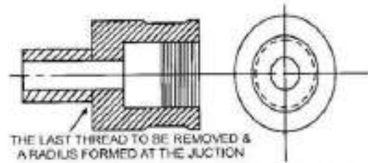
चित्र 12/70: टिपिकल माइल्ड स्टील डिस्टेंस पीस ऑफ माउंटनिंग
