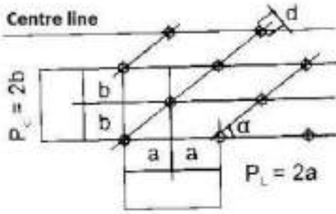
चित्र 4/13: छिद्रों का नियमित विस्मयकरण
