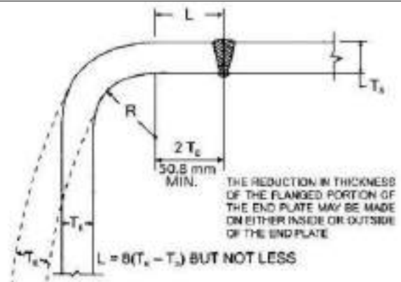
चित्र 12/8: शेल से अधिक मोटाई के प्लैज्ड एंड प्लेट्स थिककर
