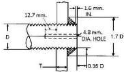
चित्र 12/48: फायरबॉक्स और कम्बस्टन चैंबर स्टेस का अटैचमेंट
