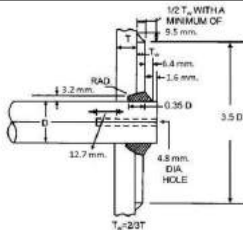
चित्र 12/52: बार स्टेस का अटैचमेंट
