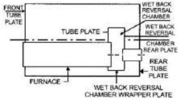
चित्र 12/26: वेट बैक बॉयलर
