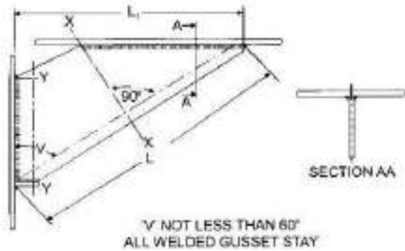
चित्र 12/101: ऑल वेल्डेड गसेट स्टे के लिए विशिष्ट ब्यौरा
