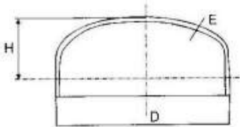
चित्र. 4/16: दीर्घवृत्ताकार हैड
