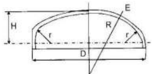
चित्र.4/17: टोरिसफेरिकल हैड
