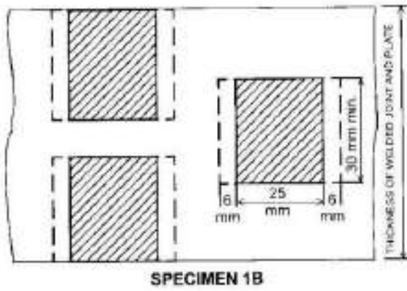
चित्र 12/74: थिक प्लेट में रिड्यूज्ड सेक्शन तन्पता नमूना
