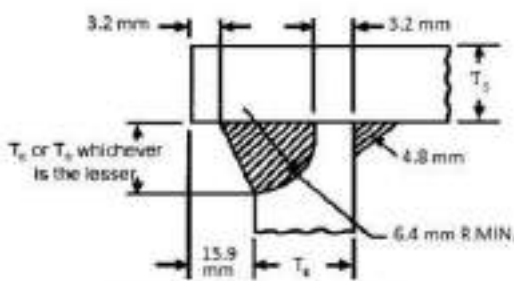
चित्र 12/12: प्लेट एंड
