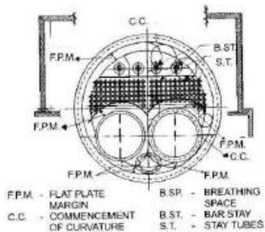
चित्र 12/90*: इकोनॉमिक बॉयलर का एंड प्लेट का टिपिकल अरेंजमेंट
