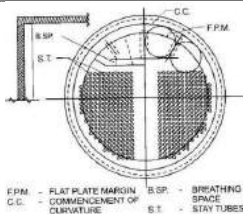
चित्र 12/92*: मल्टी ट्यूबलर बॉयलर पर एंड प्लेट का टिपिकल अरेंजमेंट
