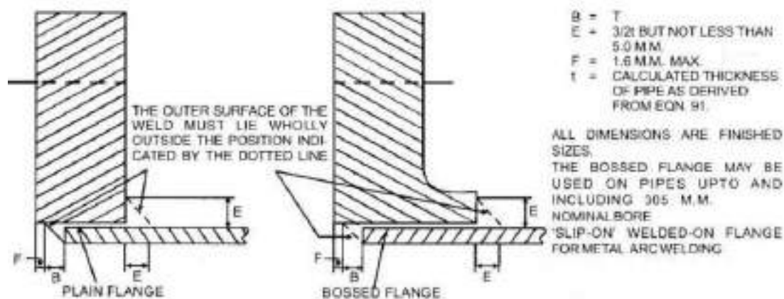
चित्र 7 / 32 : फ्लैज बोर और पाइप के ओडी के बीच निकासी के लिए [विनियम 263(2) देखें।]
