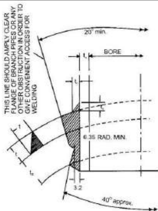
चित्र 4/30: प्रतिपूर्ति रिंग के साथ स्टैंडपाइप या ब्रान्च में वेल्ड किया
