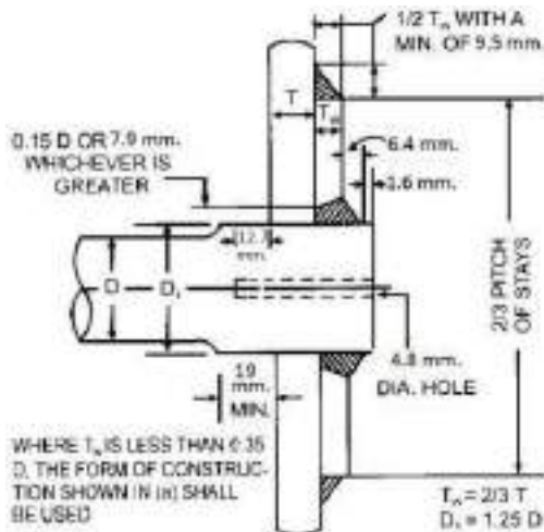
चित्र 12/59: बार स्टेस का अटैचमेंट
