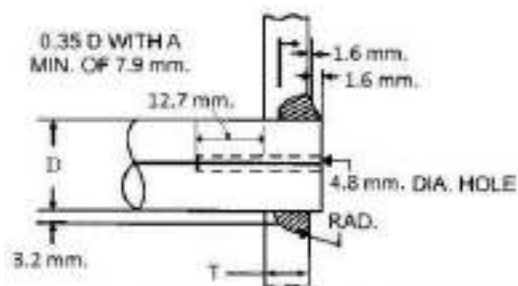
चित्र 12/49: फायरबॉक्स और कम्बस्टन चैंबर स्टेस का अटैचमेंट
