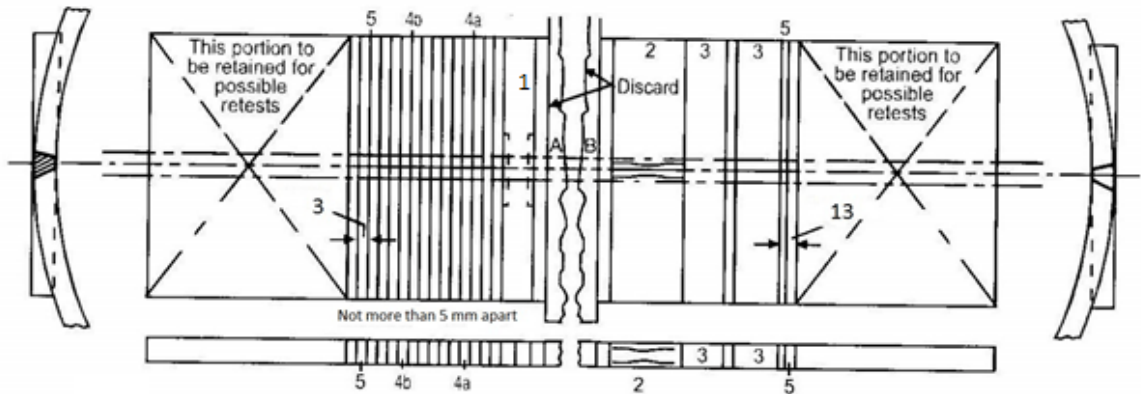
चित्र 4/1: टेस्ट प्लेट्स का विवरण
