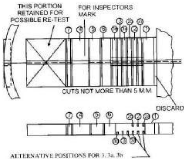
चित्र 12/71: परीक्षण प्लेट्स का ब्यौरा
