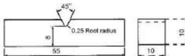
चित्र 4/7: मानक वी-नॉच टेस्ट पीस
