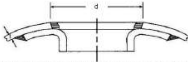
चित्र. 10/11 : अण्डाकार मेनहोल फ्लैण्ड फ्रेम वेल्डेड टू शेल
