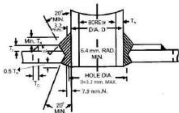
चित्र 12/112: 127 मिमी से अधिक स्टैंड पाइप्स के लिए न्यूनतम वेल्ड अटैचमेंट जिन्हें प्रतिपूरक प्लेट की आवश्यकता है
