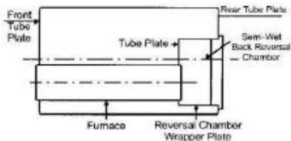
चित्र 12/28: सेमी-वेट बैक बॉयलर
