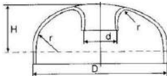
चित्र. 4/18: मैनहोल हैड (दीर्घवृत्ताकार या टोरिसफेरिकल)
