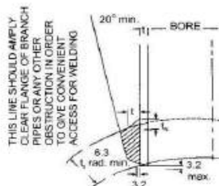
चित्र 4/32: स्टैंडपाइप या ब्रान्च में वेल्ड किया
