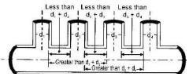
चित्र 7 / 7: विशिष्ट ब्रांच के टुकड़े
