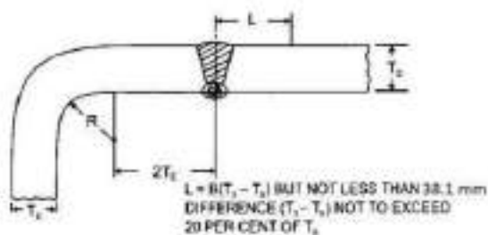
चित्र 12/10: फ्लैज्ड प्लेट एंड प्लेट्स
