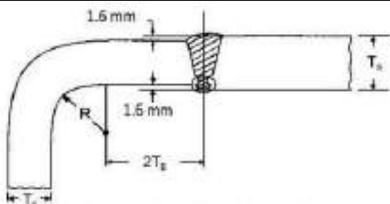
चित्र 12/11: फ्लैज्ड प्लेट एंड प्लेट्स टू शेल (एंड से अधिक मोटाई के शेल)
