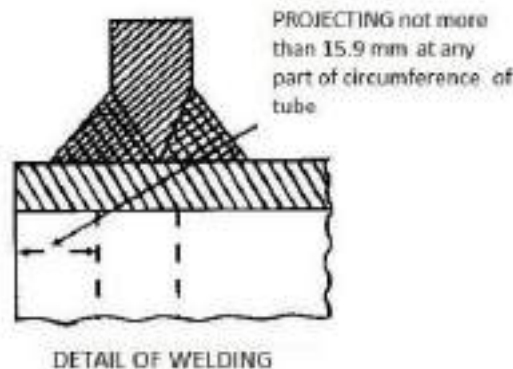
चित्र 3/5 वर्टिकल क्रॉस ट्यूब बॉयलरों के क्रॉस ट्यूब का फ्यूजन वेल्डिंग
