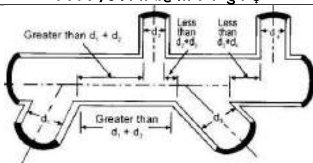
चित्र 7 /6 : विशिष्ट ब्रांच के टुकड़े
