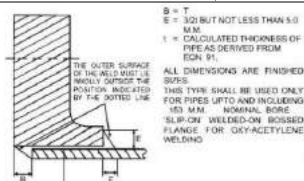
चित्र 7 / 33 : फ्लैज बोर और पाइप के ओडी के बीच निकासी के लिए [विनियम 263(2) देखें]
