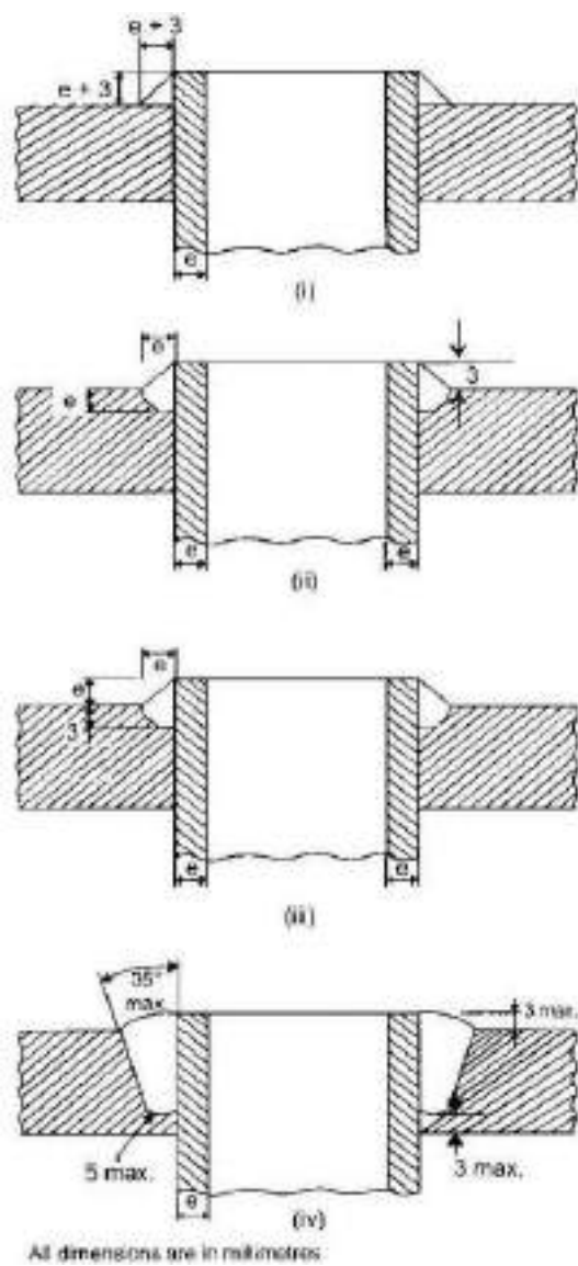
चित्र 12/84: स्टे ट्यूब का टिपिकल अटैचमेंट
