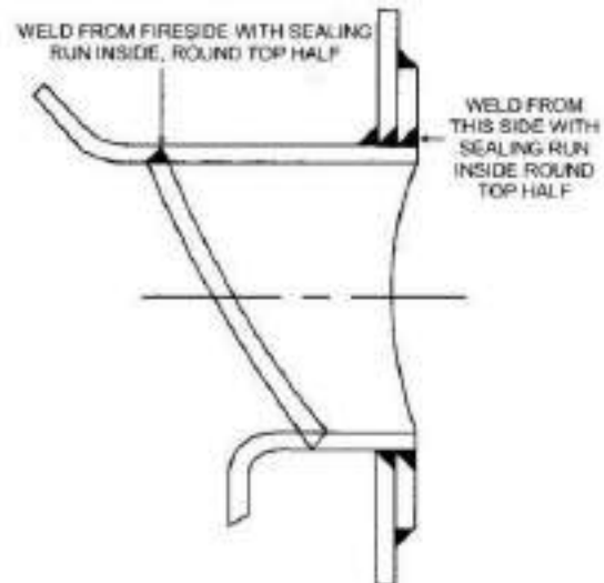
चित्र 12/41: फायरहोल माउथपीस
