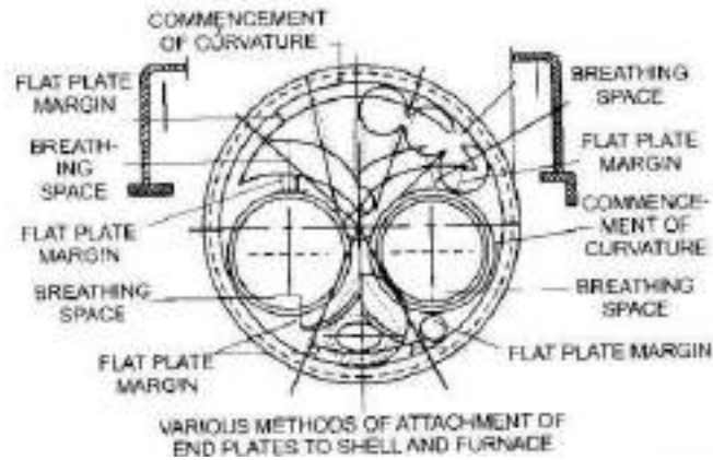
चित्र 12/86: लंकाशायर बॉयलर पर एंड प्लेट का टिपिकल अरेंजमेंट
