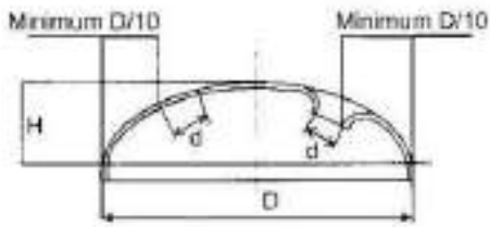
चित्र. 4/19: ओपनिंग इन हैड
