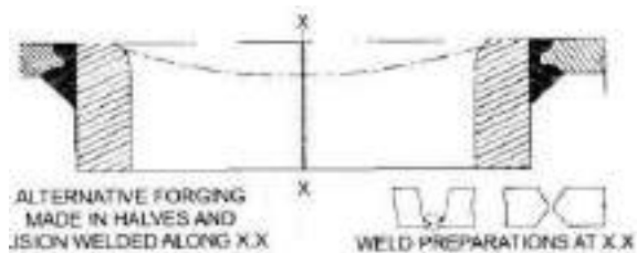
चित्र 12/65: फ्यूजन वेल्डेड ओवल मैनहोल फ्रेम
