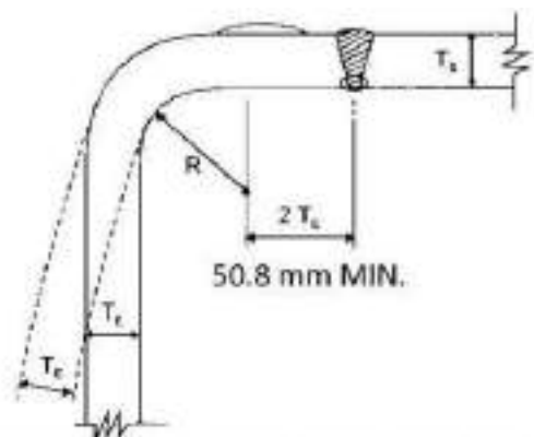
चित्र 12/9: शेल से अधिक मोटाई के फ्लैज्ड एंड प्लेट्स
