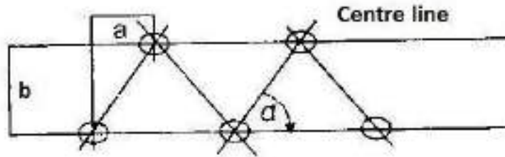
चित्र 4/15: छिद्रों का नियमित सॉ-टूथ पैटर्न
