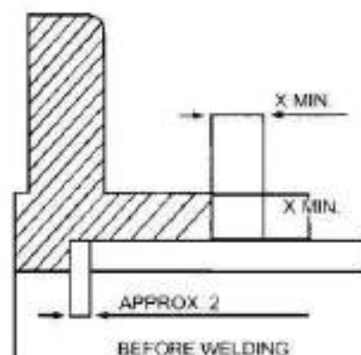
चित्र 7 / 32 : फ्लैज बोर और पाइप के ओडी के बीच निकासी के लिए [विनियम 263(2) देखें।]
