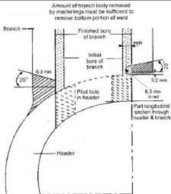
चित्र 4/33 हैडर पर आंतरिक मशीनरी के साथ जोड़ा गया हिस्सा
