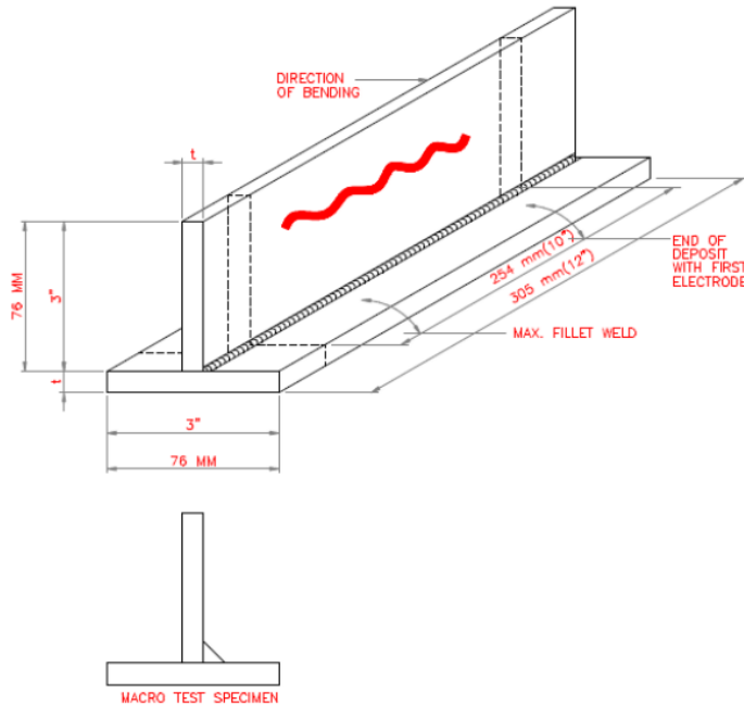
चित्र 13/5: प्रदर्शन योग्यता के लिए फिलेट वेल्ड साउंडनेस परीक्षण
