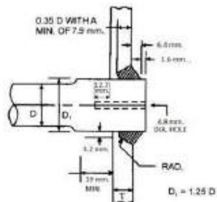
चित्र 12/51: बार स्टेस का अटैचमेंट
