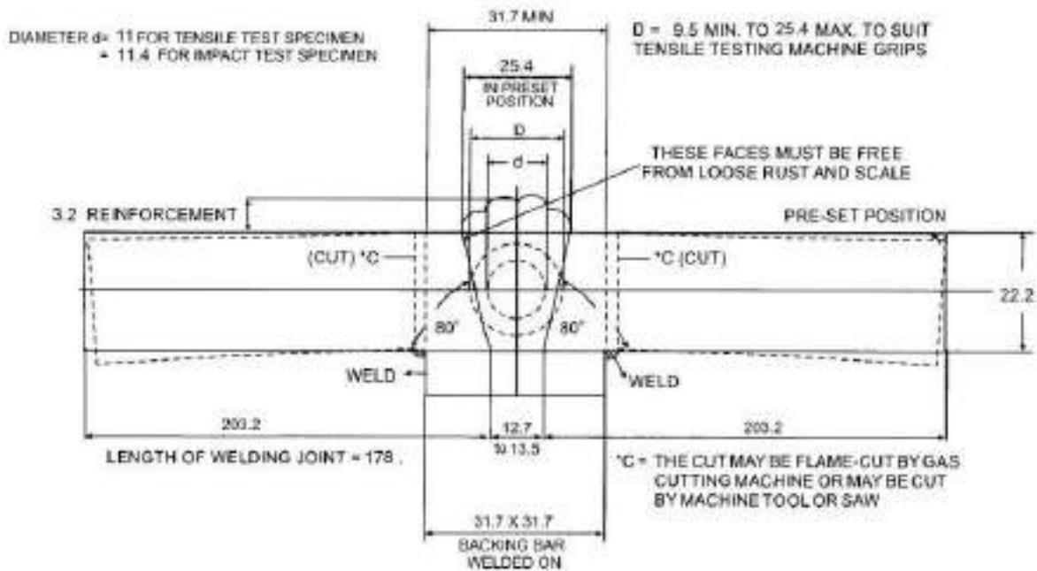
चित्र 2/2: ऑल-वेल्ड मेटल परीक्षण नमूनों को तैयार करने की पद्धति
