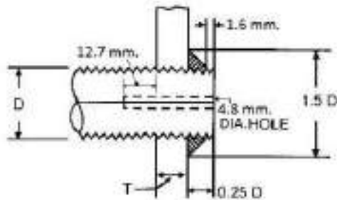
चित्र 12/47: फायरबॉक्स और कम्बस्टन चैंबर स्टेस का अटैचमेंट
