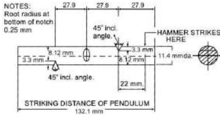
चित्र 2/4: प्रभाव परीक्षण नमूना
