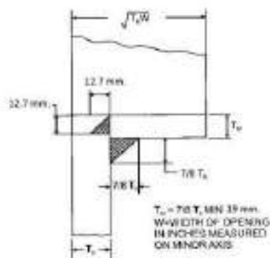
चित्र 12/68: प्लेट एंड प्लेट में मैनहोल के लिए वेल्डिंग ब्यौरा
